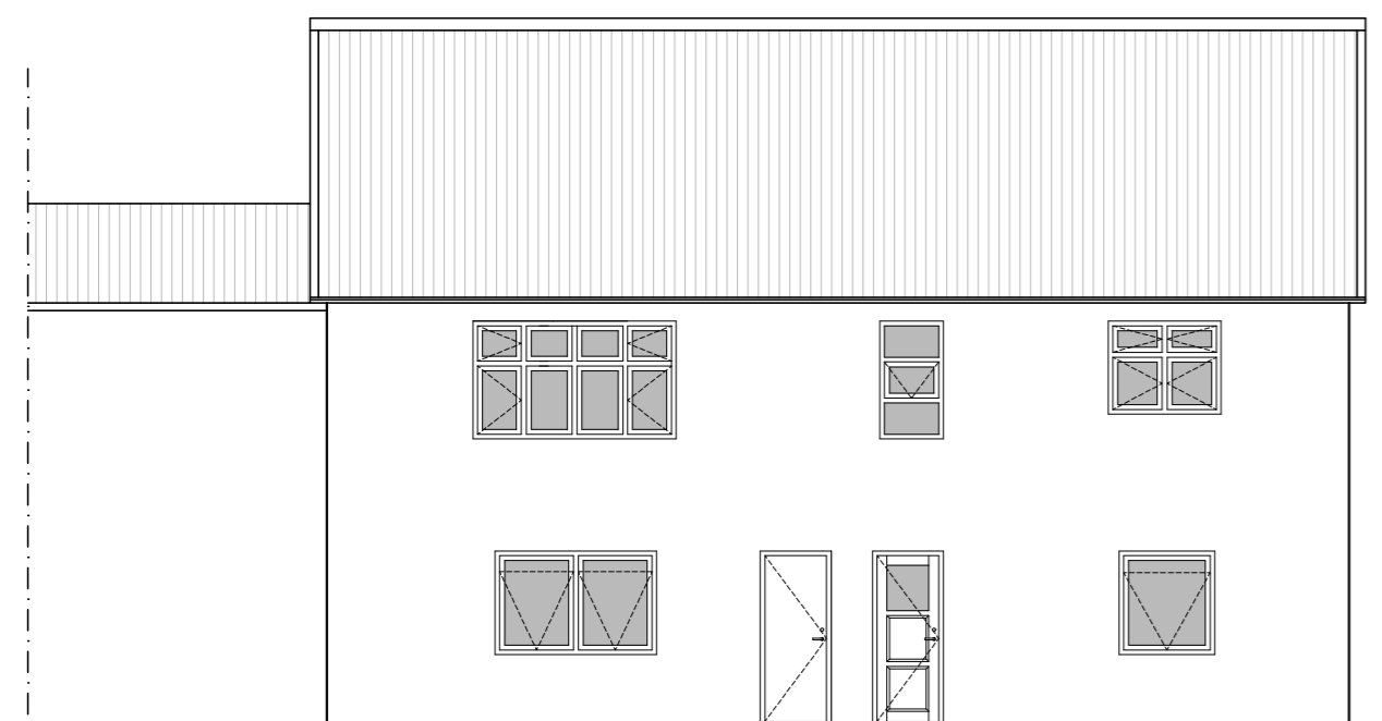
AUSTUR 1:100
